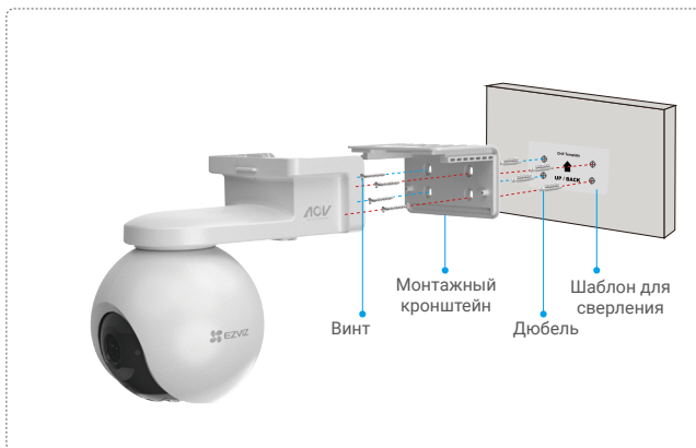
Рисунок 2. Монтаж на стену
