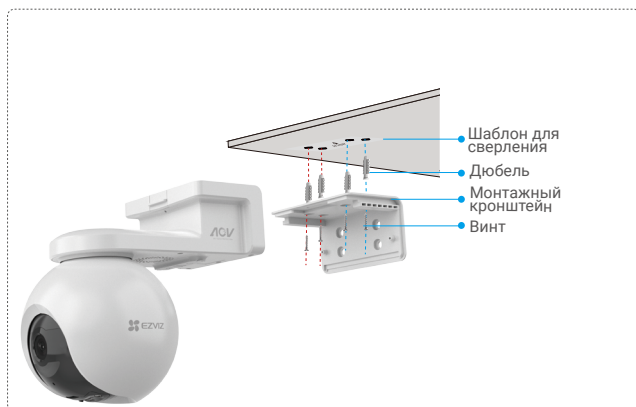
Рисунок 1. Монтаж на потолок
